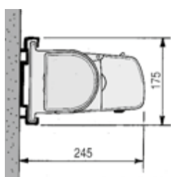
Staffe attacco parete/soffitto
