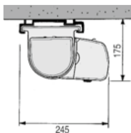
Staffe attacco parete/soffitto
