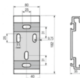
Staffa attacco parete/soffitto
