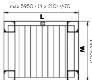
max dimensions single module
